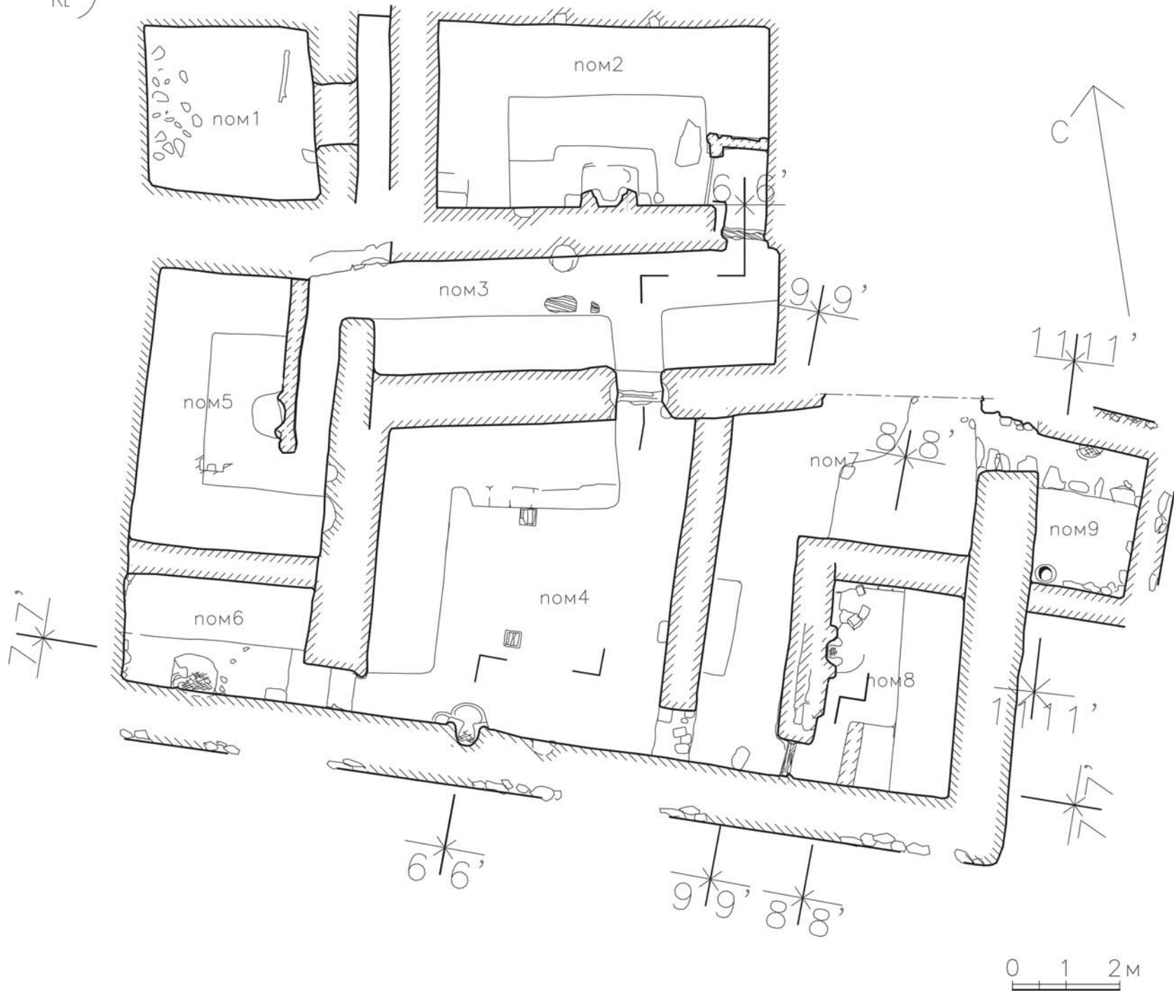
11. Шахристан, усадьба 1. План Е.Н. Буклаевой
