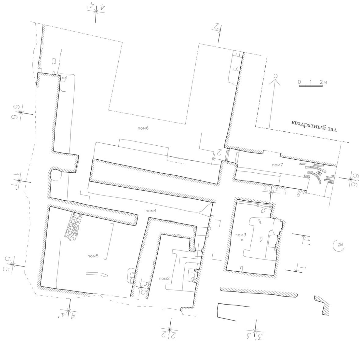
32. План раскопанного участка Цитадели II. (И.О. Гуров, Е.Н. Буклаева)
