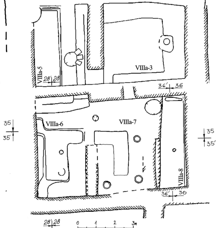
Дом VIIIa. План, архитектурные разрезы.
